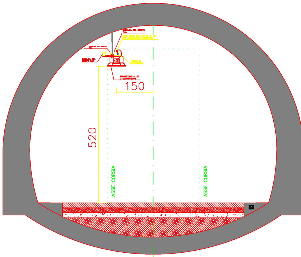
Fig1 - Sezione caratteristica Galleria PIANACCE
